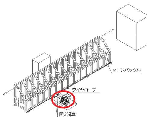
▲門開閉例
