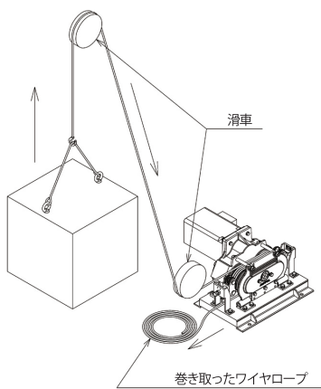
▲吊り下げ例
