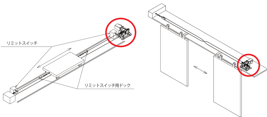
▲台車横行例
